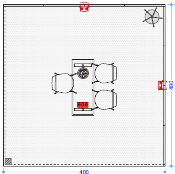
PIANTA GENERALE - MODULO 4X4 ANGOLARE
